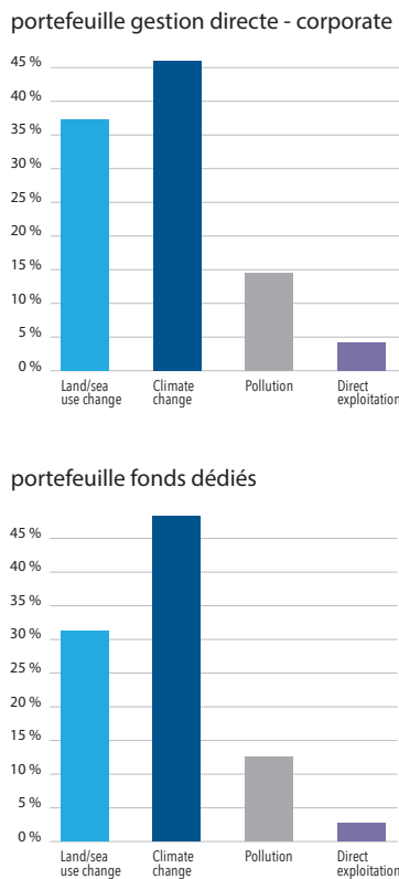
Figure 32 : Répartition par pression IPBES du score global
