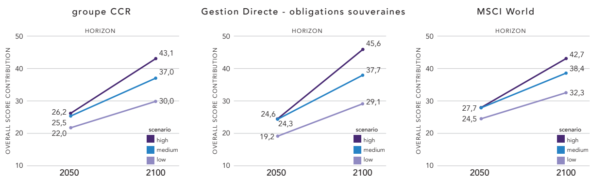
Figure 29 : Résultats de l'évaluation du risque physique selon les trois scénarios
